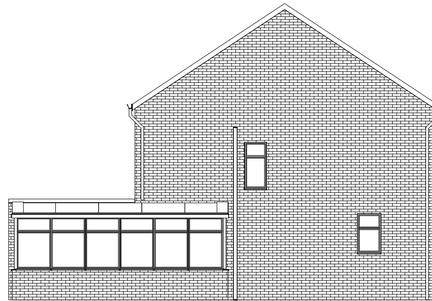
2 Side Elevation a-a 1 : 100
