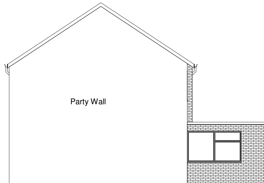
4 Side Elevation b-b 1 : 100
